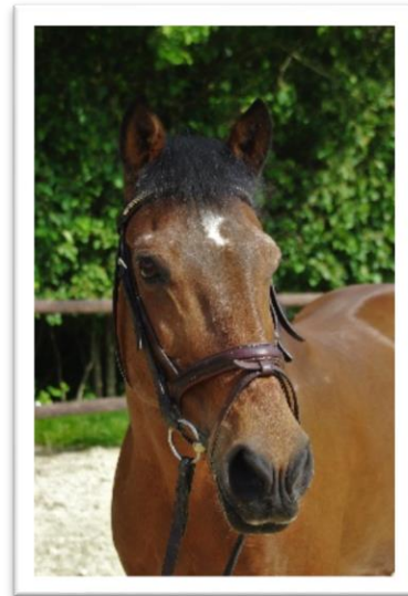
Felix
